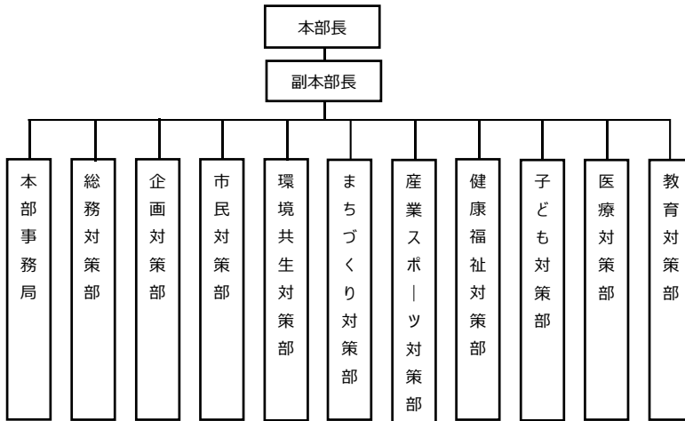
【災害対策本部組織図】
