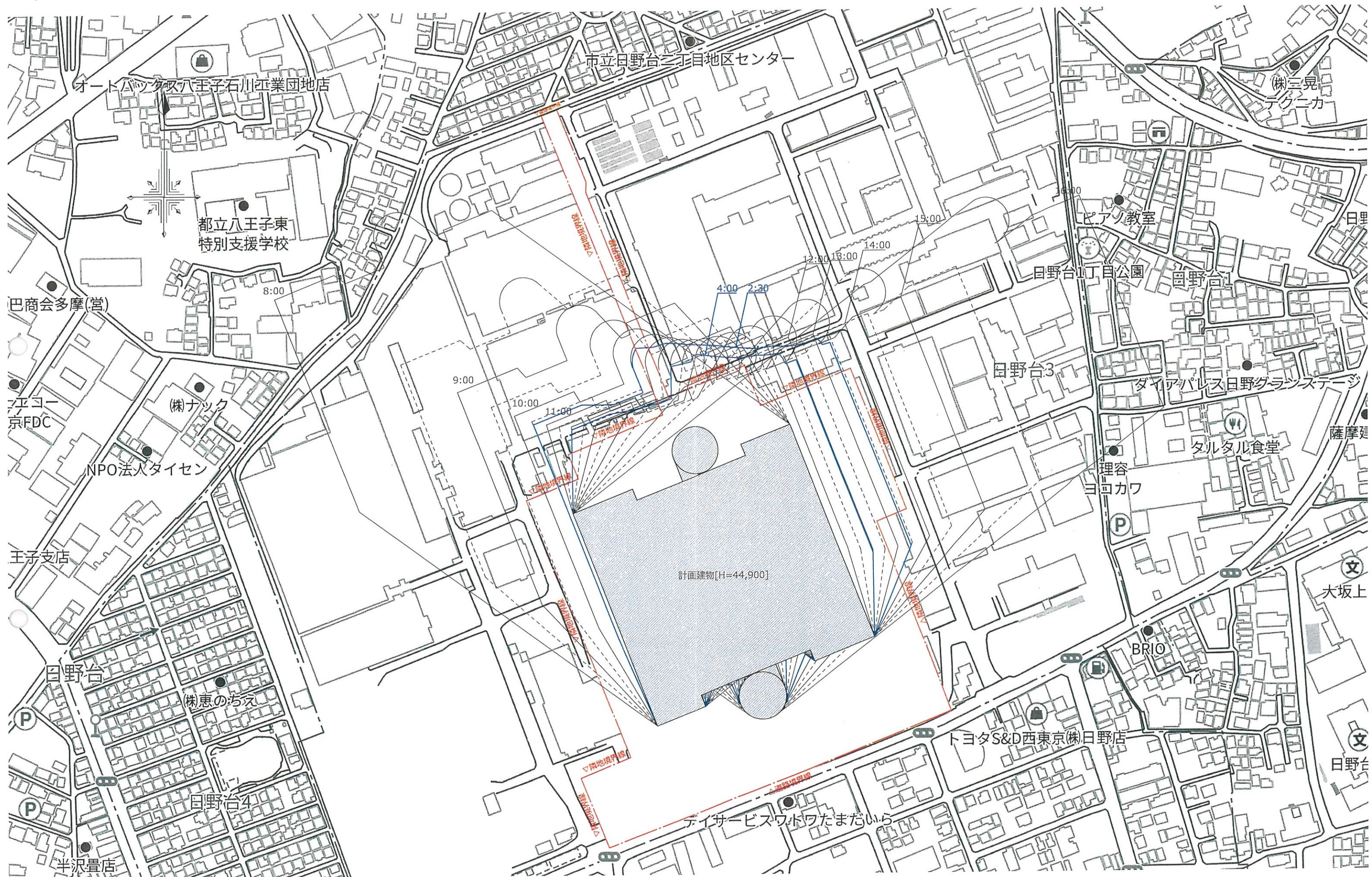
日影図 (S=1/3,000) ※等時間日影図 測定高さ 1.5m (冬至日影)
