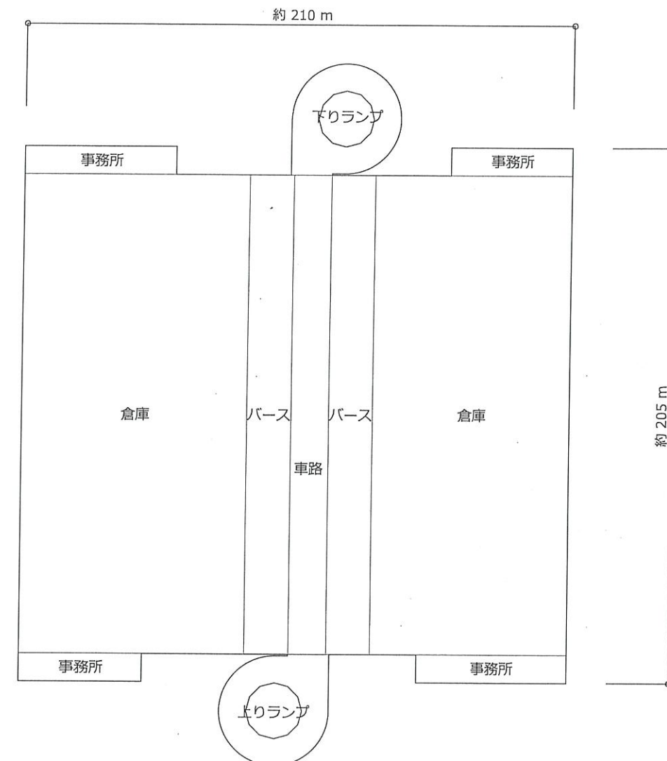
2-6階平面図 (S=1/2,000)
