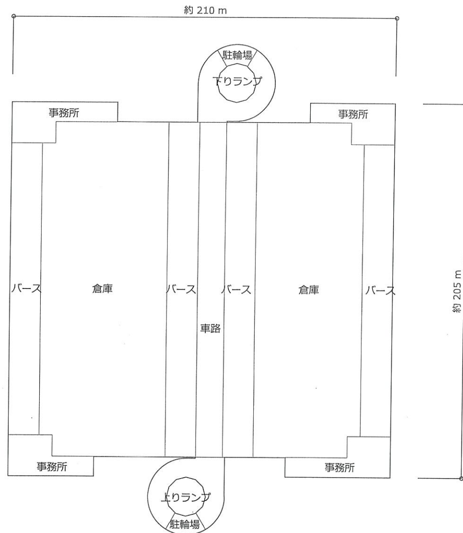
1階平面図 (S=1/2,000)
