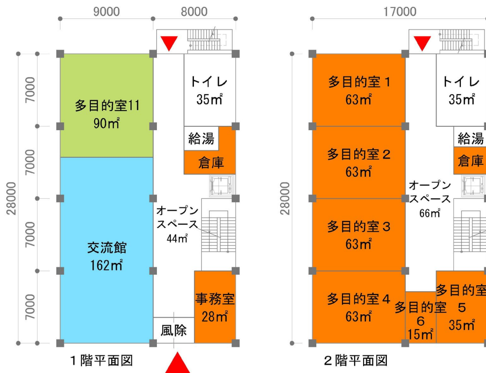
図 3.9 敷地 B 複合施設平面計画（モデルプラン）
