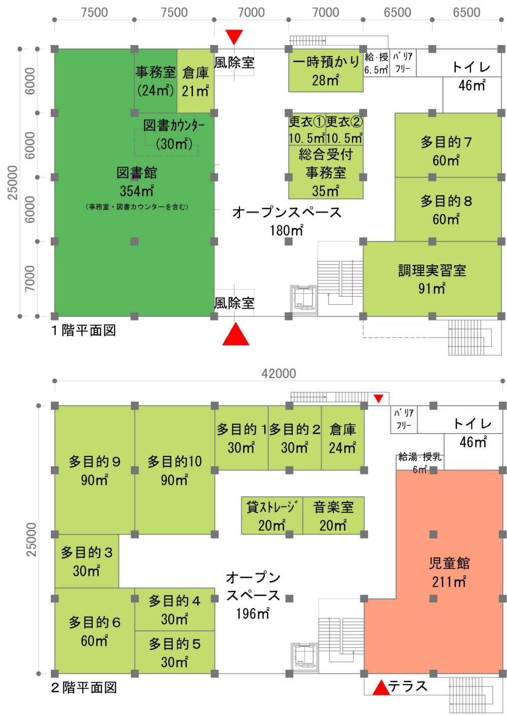
図 3.7 敷地 A 複合施設平面計画（モデルプラン）
