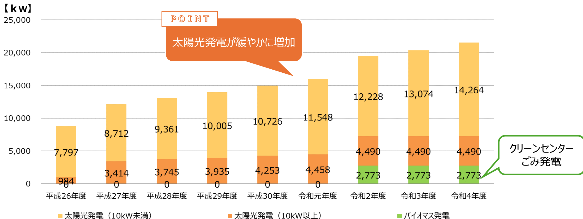
区域の再生可能エネルギーの導入設備容量の推移（累積）
