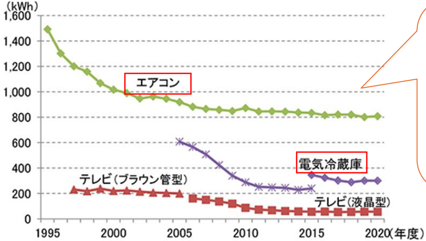
【主要家電製品のエネルギー消費効率の変化】
