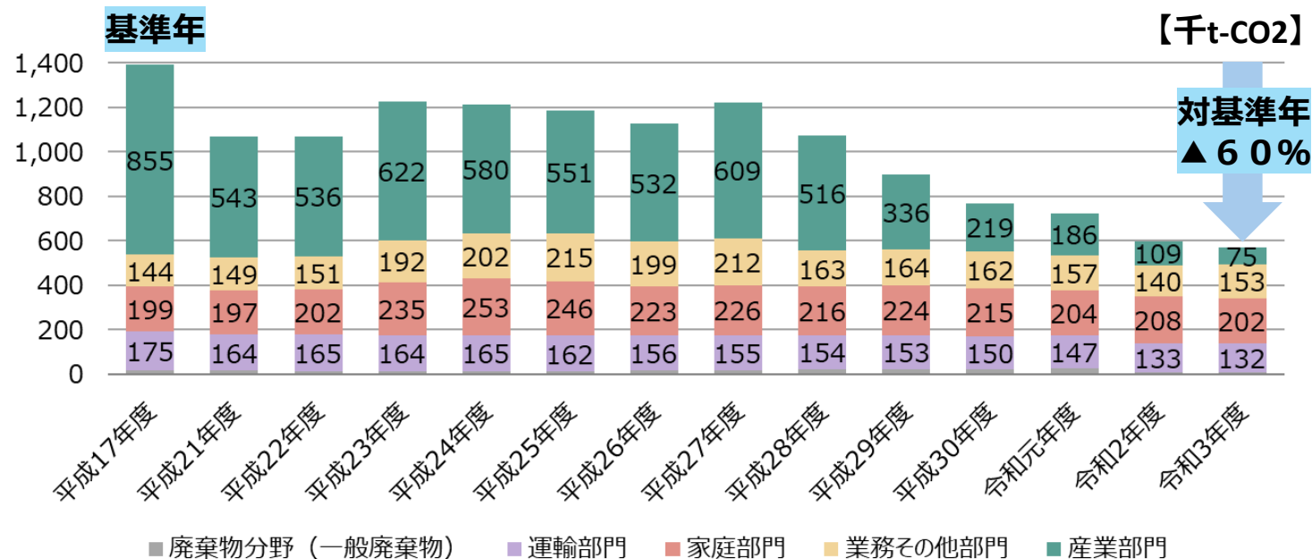
日野市の部門・分野別CO 2 排出量の推移
