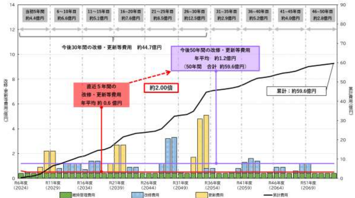
図 7-2 対策後の改修・更新等費用の推計
