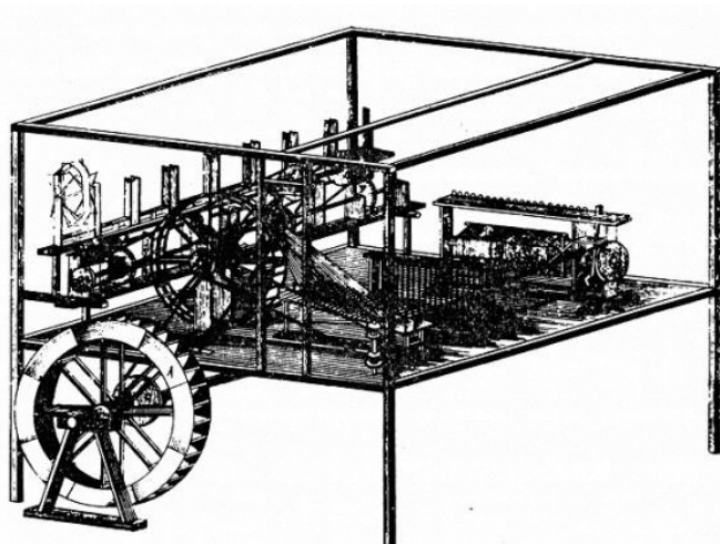
水車使用八丁撚糸機図 正田健一郎編『八王子織物史』上巻
