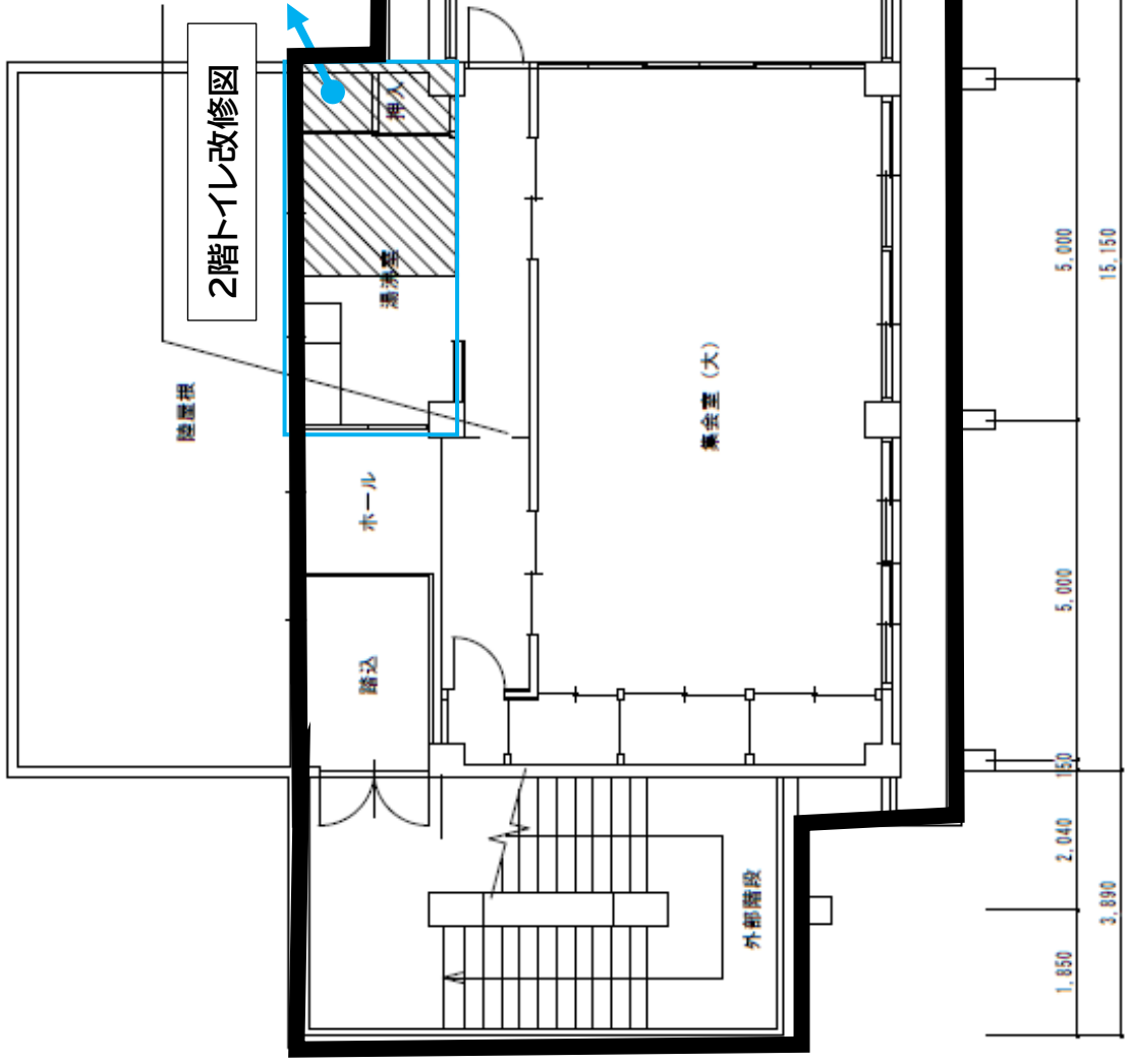
平面図 2階
