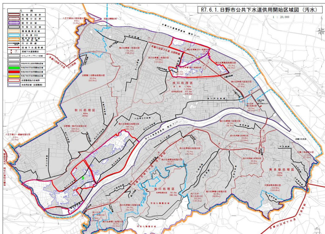
図 30 日野市公共下水道供用開始区域図（污水）（令和 7 年 6 月 1 日時点） 【第 72 回都市計画審議会（第 4 回検討）資料 P.4 5】
