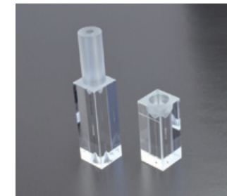
▲医療機器向けの光学フローセル。細胞の大きさ、構造を解析できる
