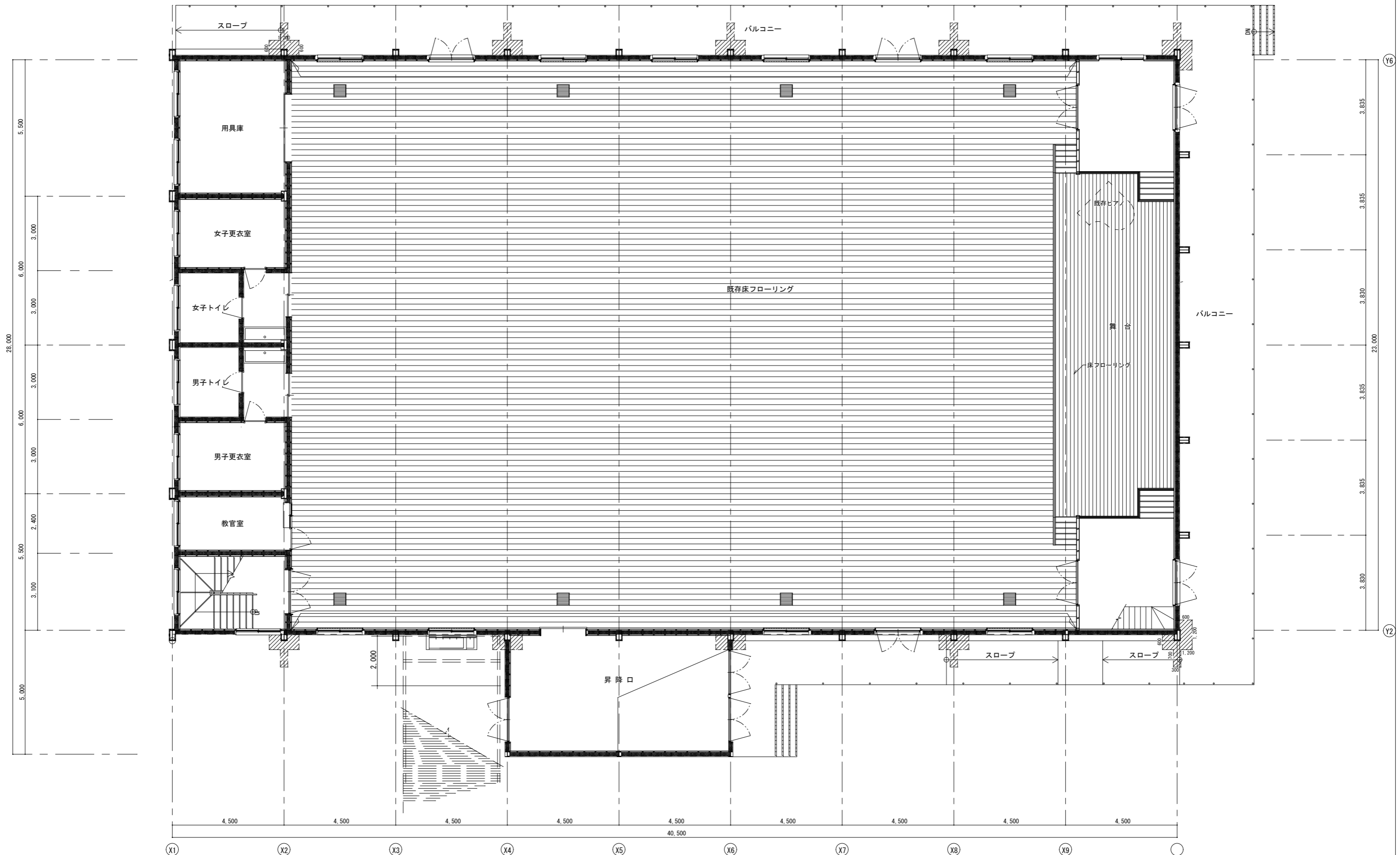
参考平面図
