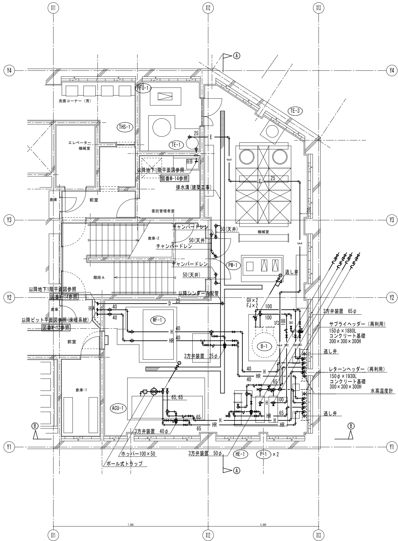
地下1階機械室詳細図 (配管)
