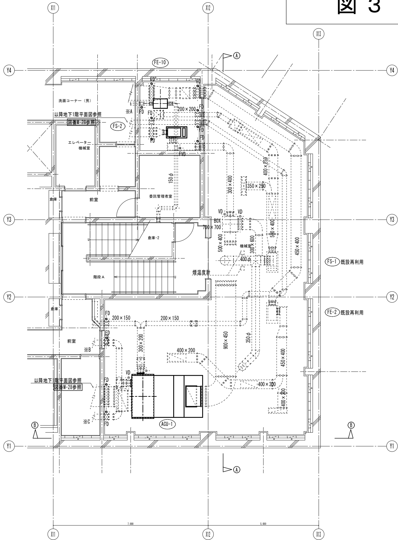
地下1階機械室詳細図 (ダクト)
