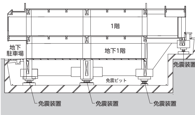
▲建物基礎の下を掘削し免震装置を取り付け
