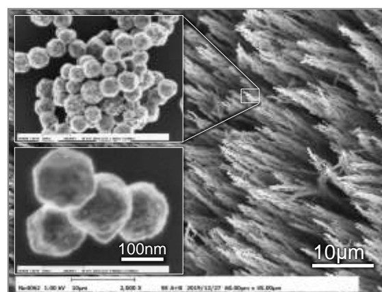
図2 高結晶性 Ni ナノ粒子のナノトラス構造
