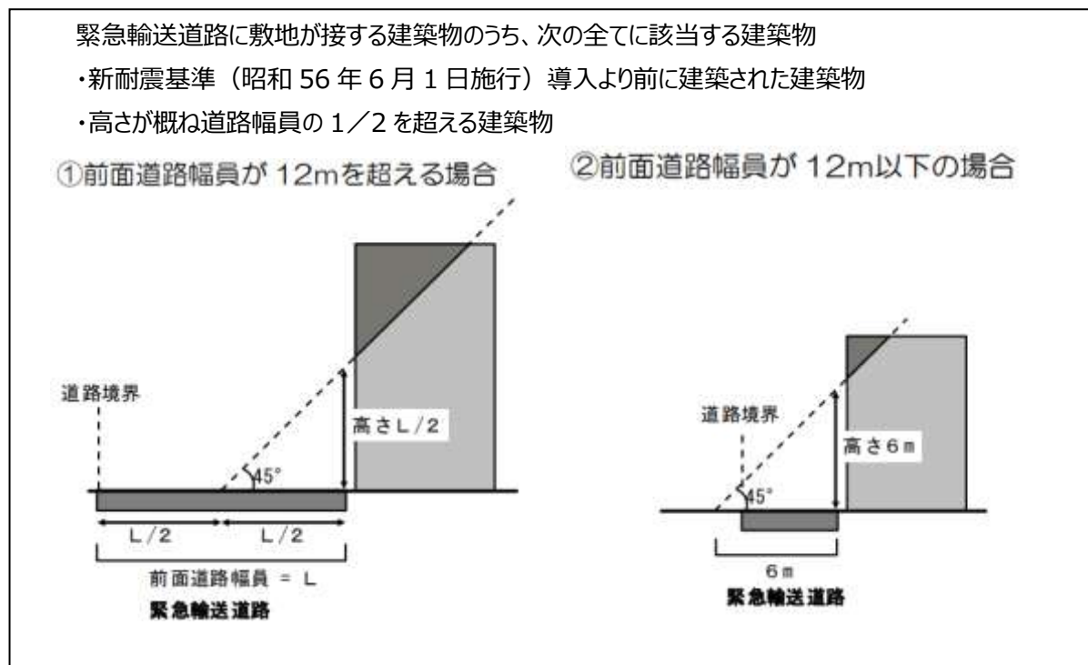
図 3 緊急輸送道路沿道建築物の定義
