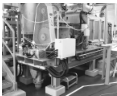
▲汚泥脱水機
