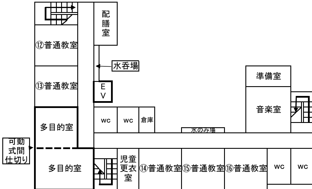
四階 平面図
