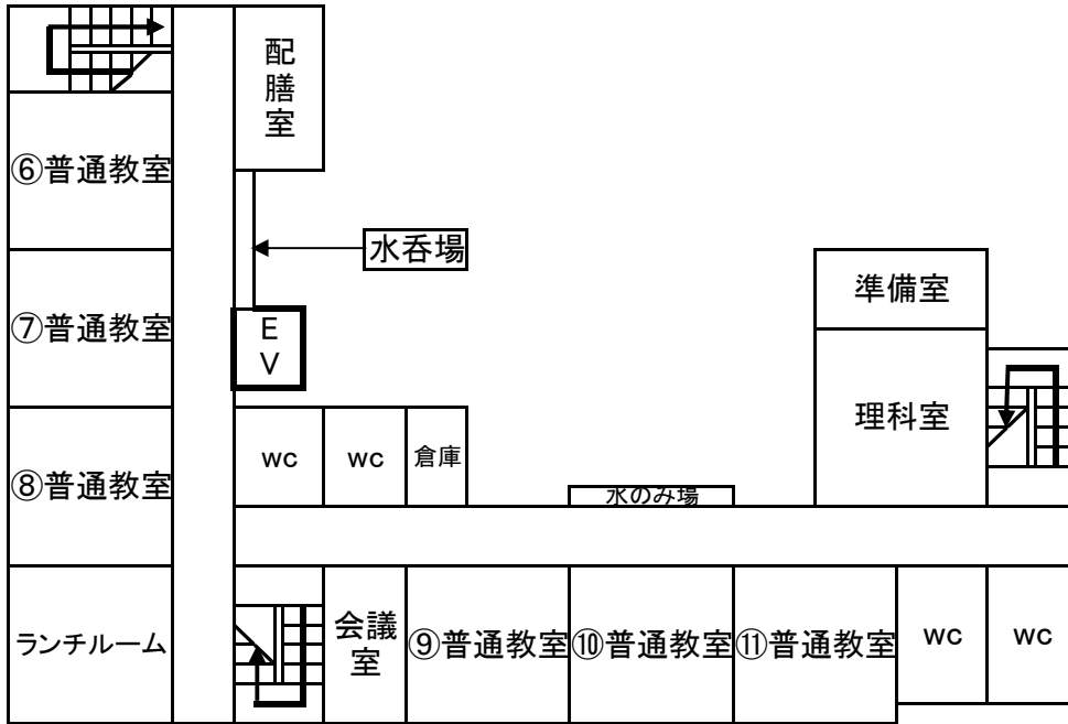
三階 平面図
